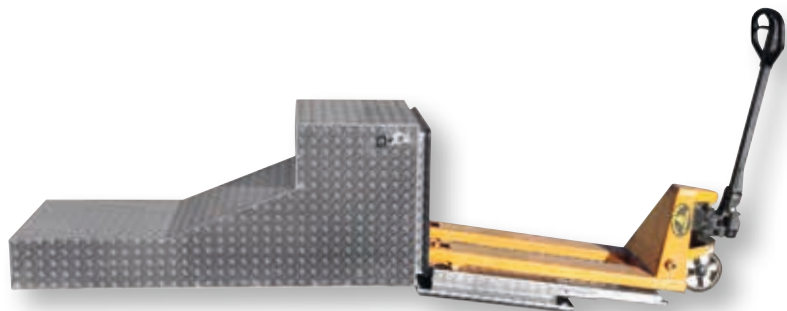
Hubwagenkasten aus Aluminium-Riffelblech mit Klappdeckel. Der Kasten ist mit Spannbügelverschlüssen gesichert und hat eine im Deckel integrierte ausziehbare Auffahrrampe für den Hubwagen.
